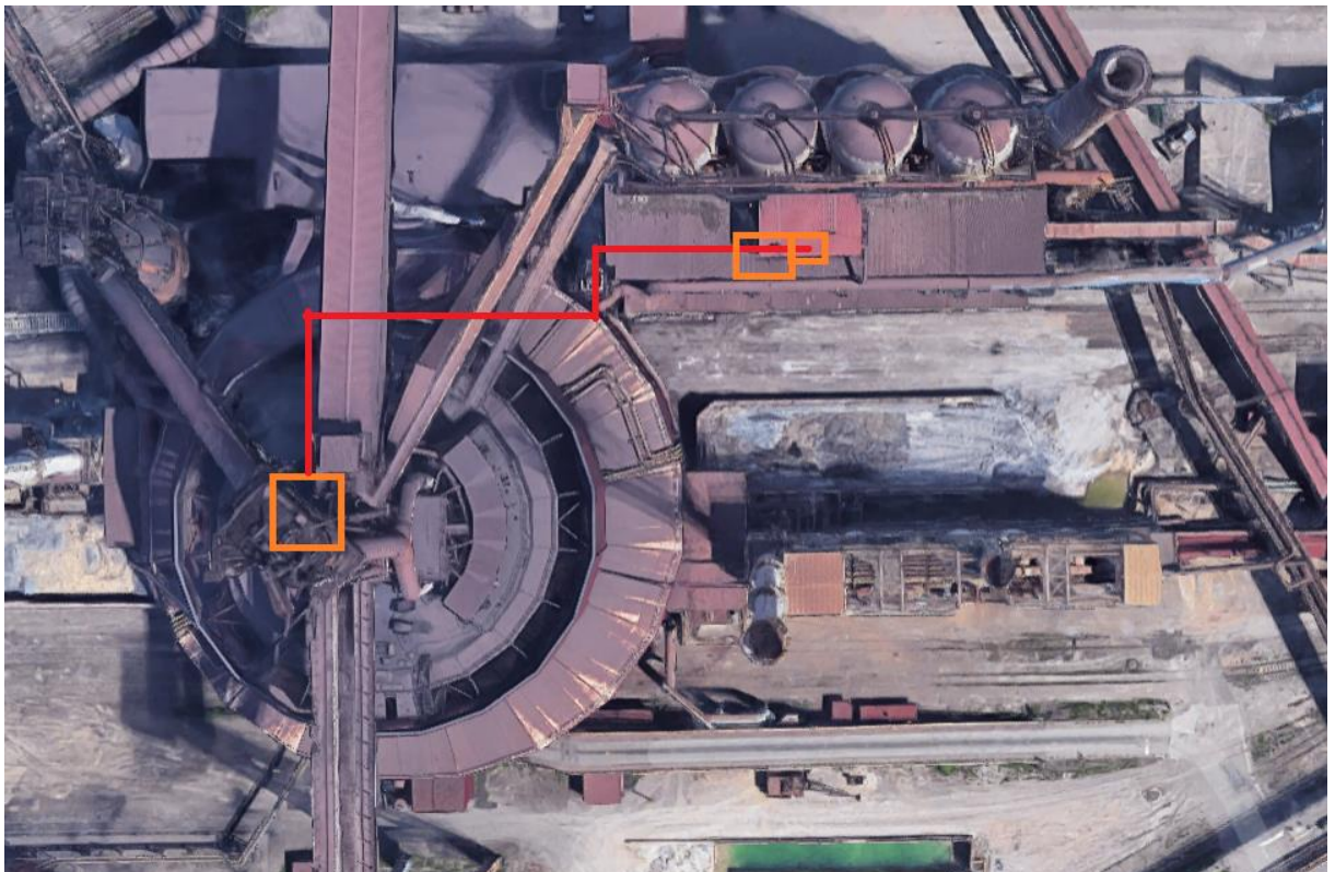
Rys. Zakładana trasa kablowa do zasilania urządzeń na podpięciu - około 150m
